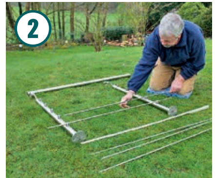
Die Rundstäbe ( \varnothing 10 mm) durch die Rundstabhalter an den Stützen schieben.
