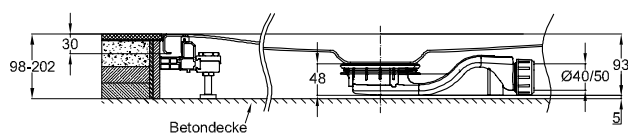
Darstellung mit Ablaufgarnitur BetteSolid 30 - 0,6 l/s, seitlicher Entwässerung, Stauhöhe 30 mm
