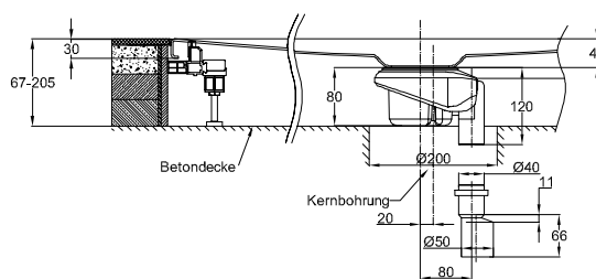
Darstellung mit Ablaufgarnitur BetteDown - 0,6 l/s, senkrechte Entwässerung, normgerechte Stauhöhe 50 mm
