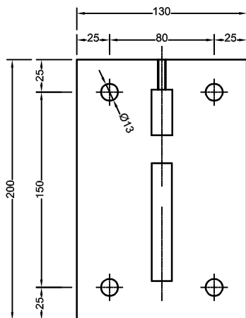
Detail Wandanschlußplatte
