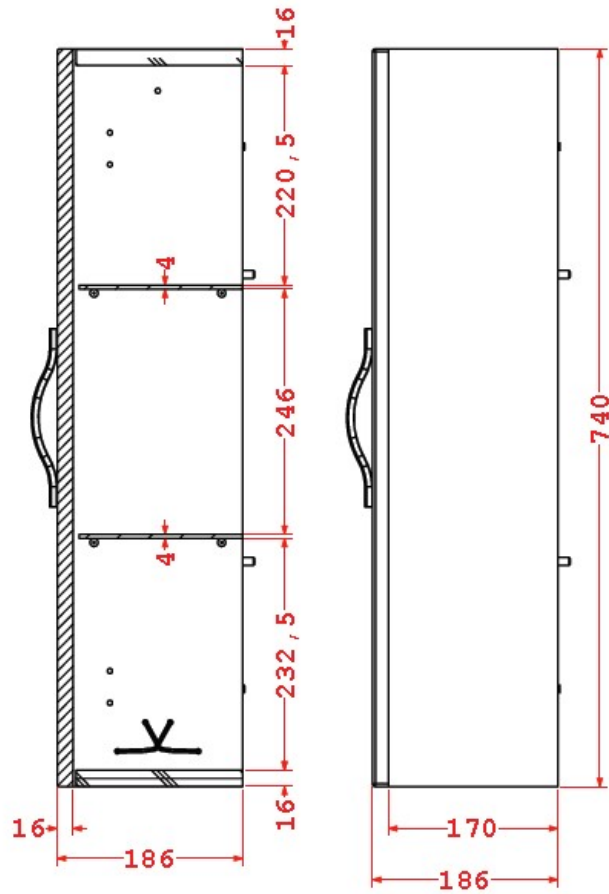
SEZIONE A-A
