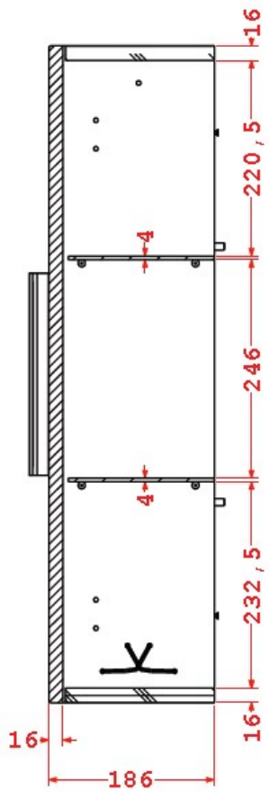
SEZIONE A-A
