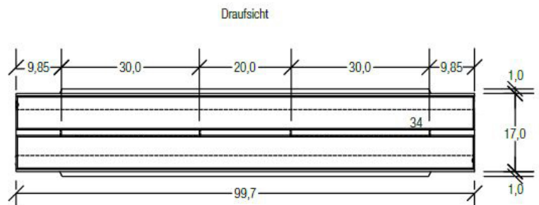
Rinne mit unterbrochenem Schlitz
