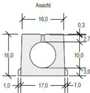
Rinnenoberfläche eben
