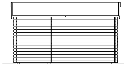
Grundriss, Schnitt und Ansichten M 1:100
