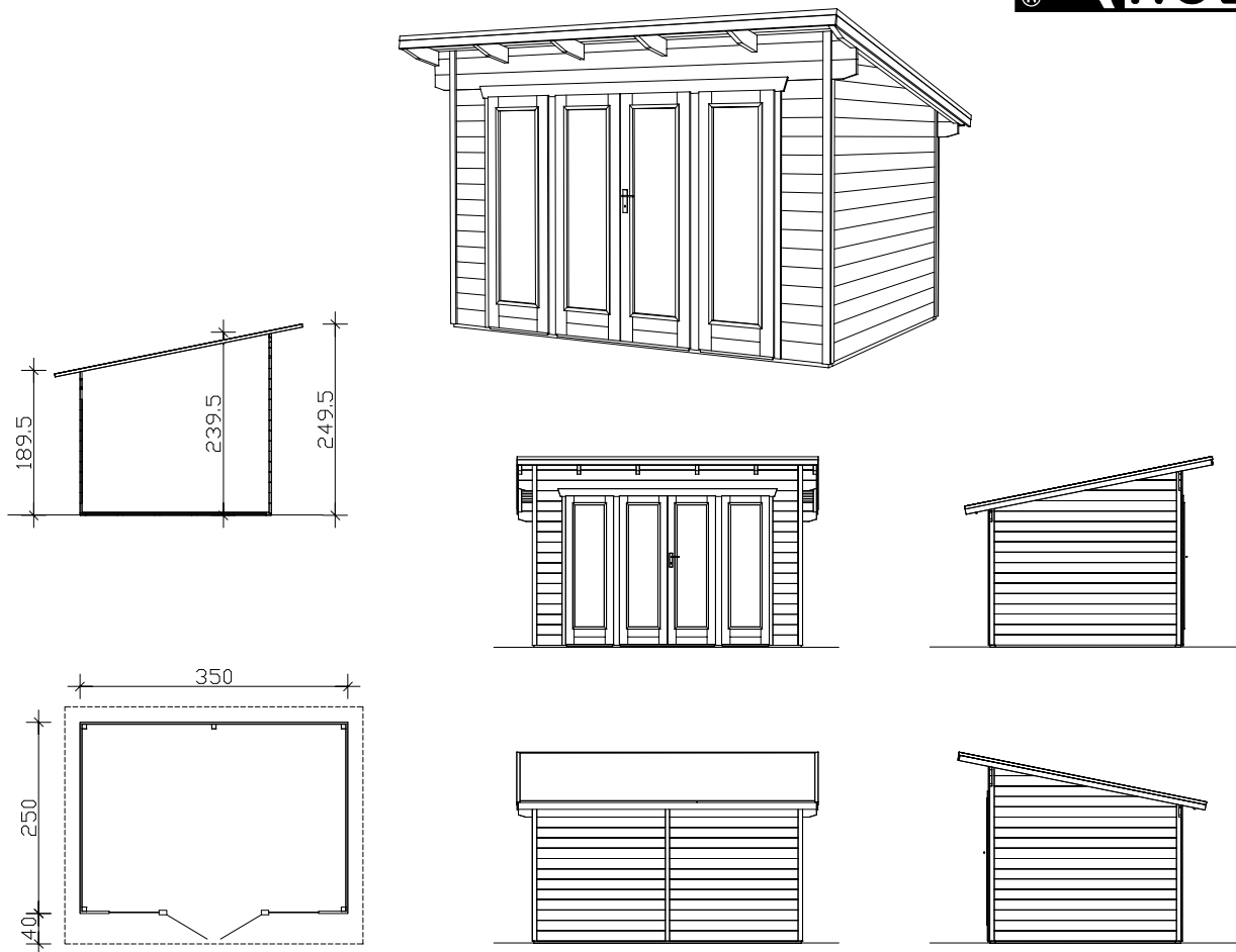
Grundriss, Schnitt und Ansichten M 1:100
