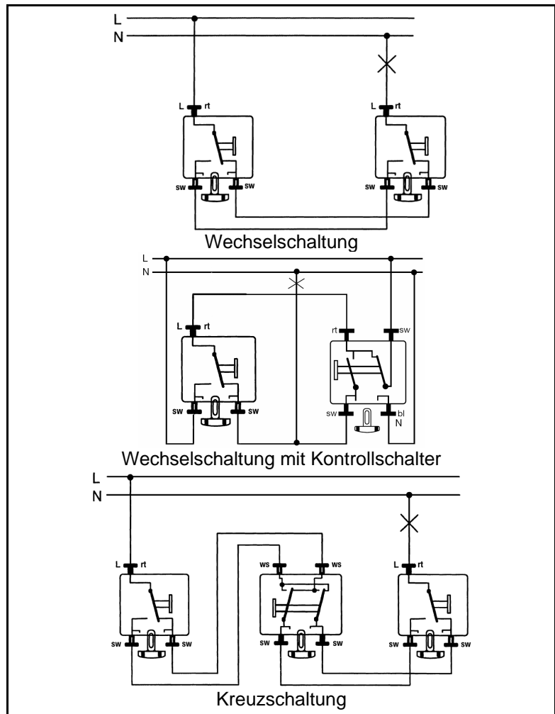
Anschlussbeispiel 506 U
