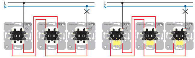
Bild 1: Kreuzschaltung / Kreuzschaltung beleuchtet: Glimmaggregat leuchtet bei „Aus“
