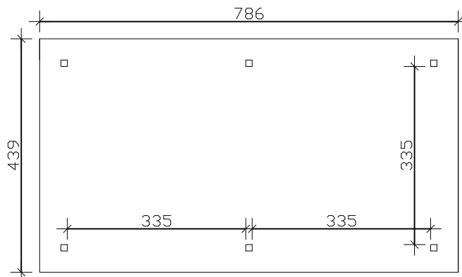
Grundriss (Gr.2)
