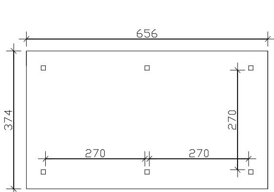
Grundriss (Gr.1)
