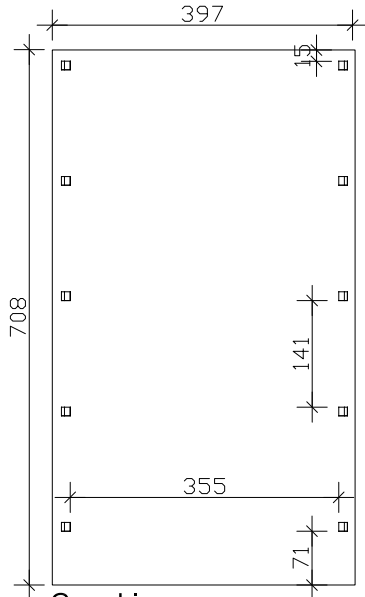
Grundriss
